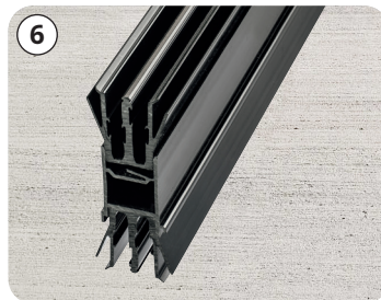
Rohrmaß 30x80 mm
